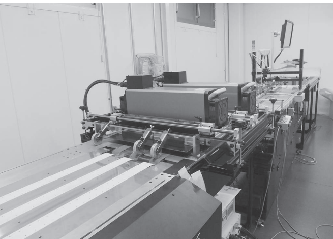
両面宛名印字機「MPS2000D」
